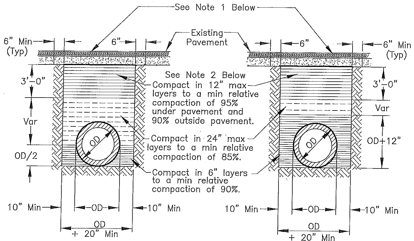
RIGID CONDUIT
